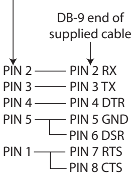
DIN to DB-9 Cable
